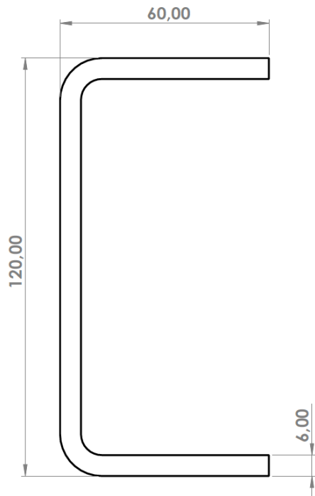
Longitudinal C 120/60/6 mm S355MC
