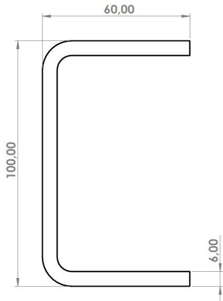
Longitudinal C 100/60/6 mm S355MC
