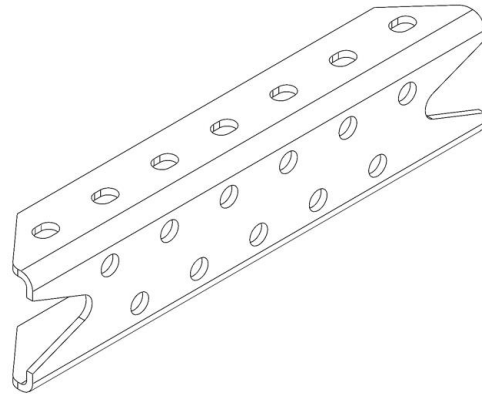
Longitudinal connector 100-5 mm S355MC
