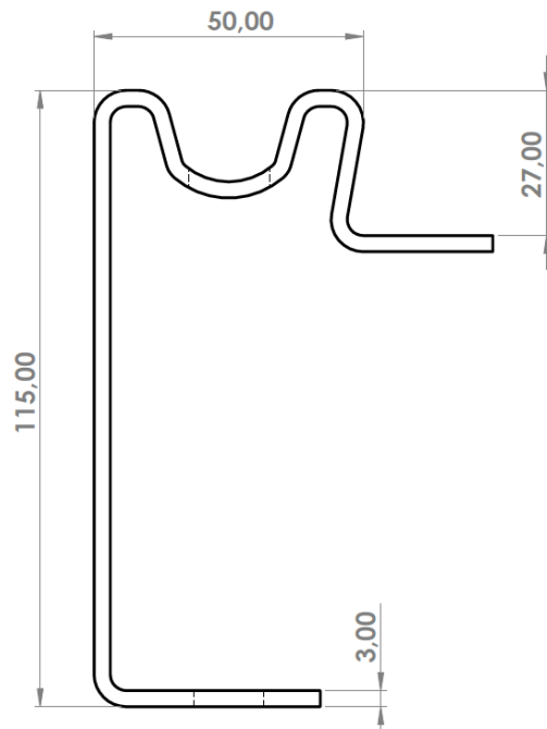
Obvodový Profil Typ UL 115/27/3 mm S355MC
