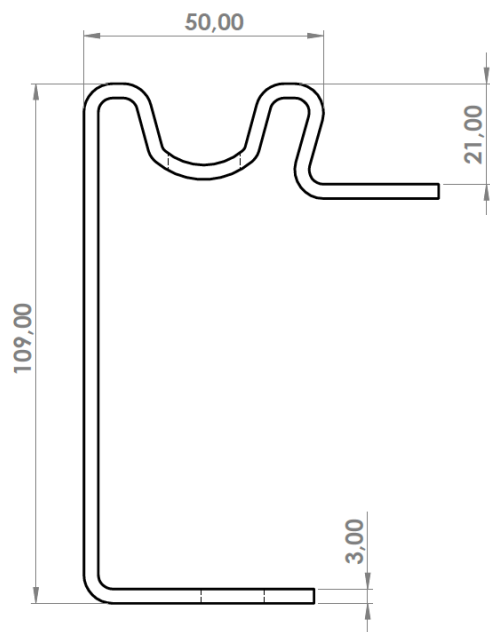
Obvodový Profil Typ UL 109/21/3 mm S355MC
