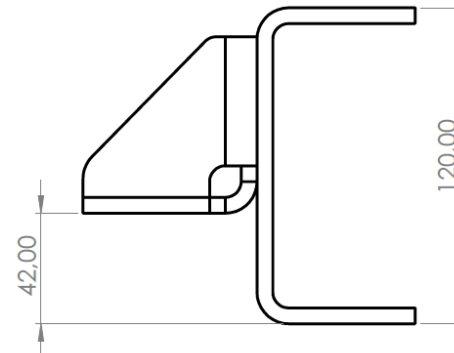
Konzole 135x67-6 mm horní poloha
