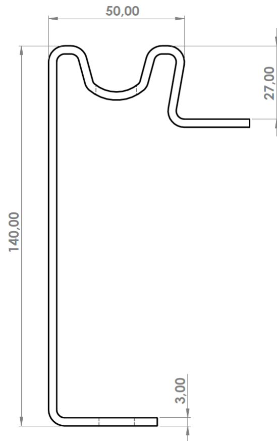
Obvodový Profil Typ UL 140/27/3 mm S355MC
