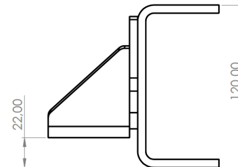
Konzole široká 218x90-6 mm
