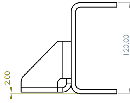
Konzole 135x67-6 mm dolní poloha
