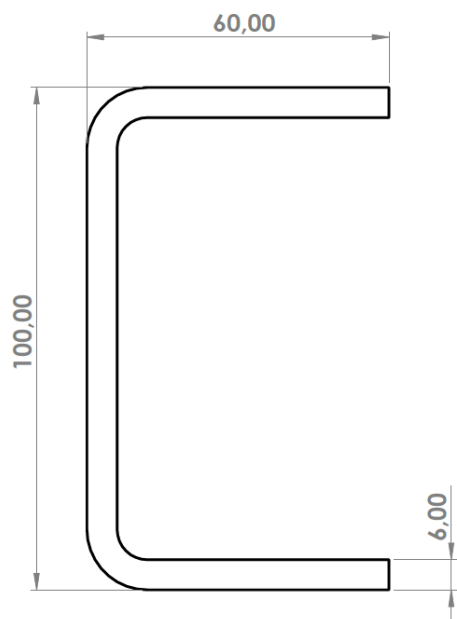
Podélník C 100/60/6 mm S355MC
