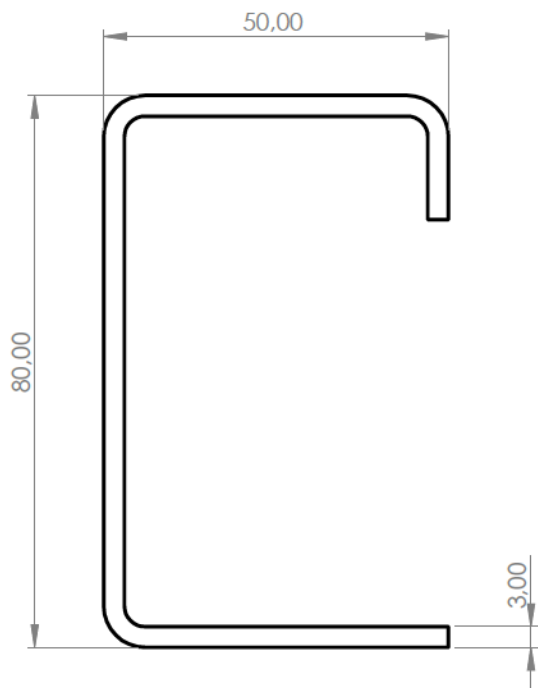
Příčník 80x50x3 mm S355MC
