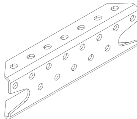
Spojka podélníku 120-5 mm S355MC
