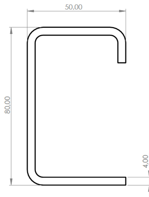
Příčník 80x50x4 mm S355MC
