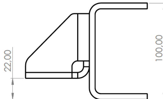
Konzole 135x67-6 mm
