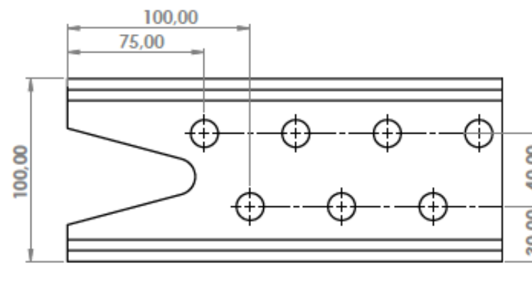
Spojka podélníku 100-5 mm S355MC
