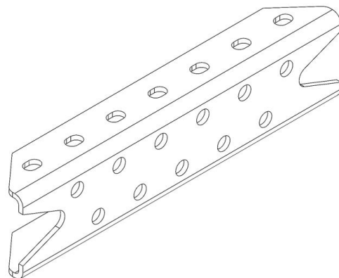
Spojka podélníku 100-5 mm S355MC
