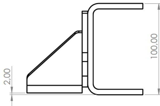
Konzole široká 218x90-6 mm
